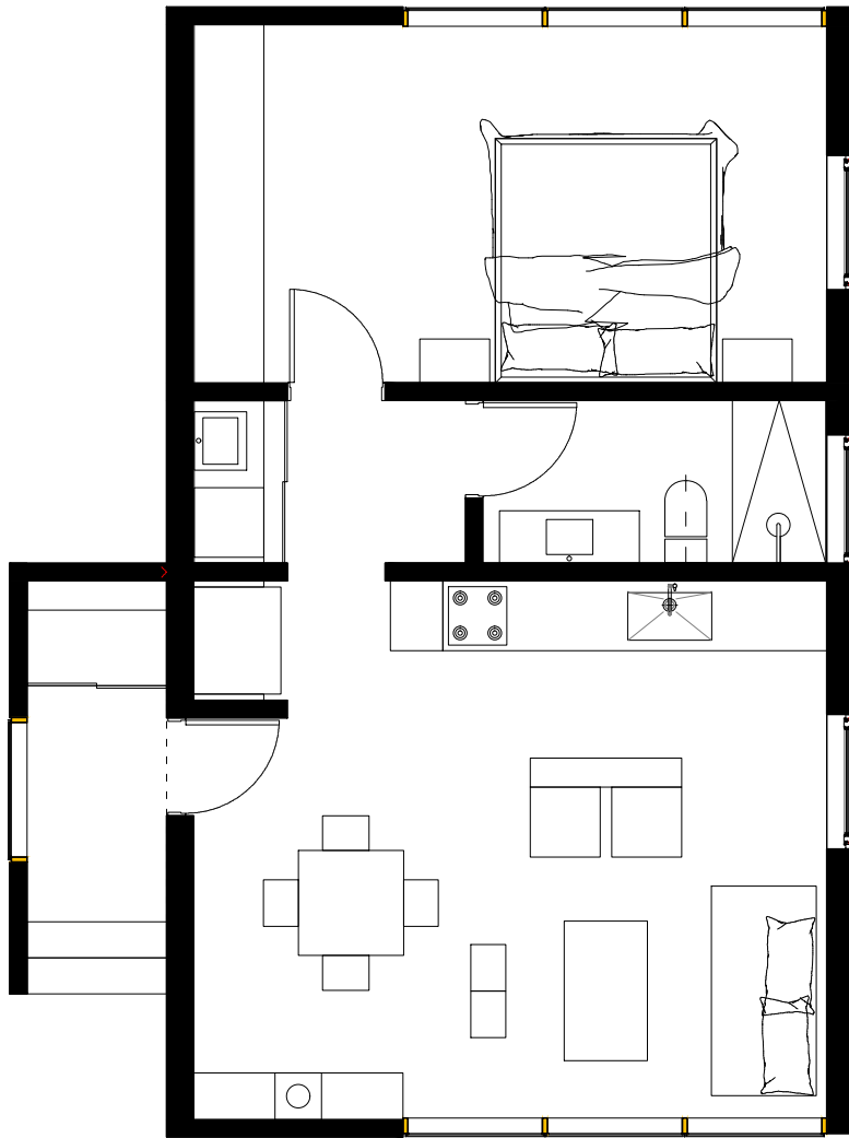
NOKI 2 _ 65 PLANTA
