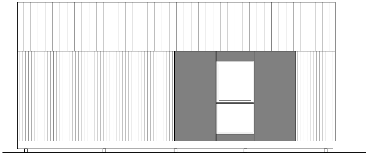
NOKI 2 _ 65 ELEVACION 2
